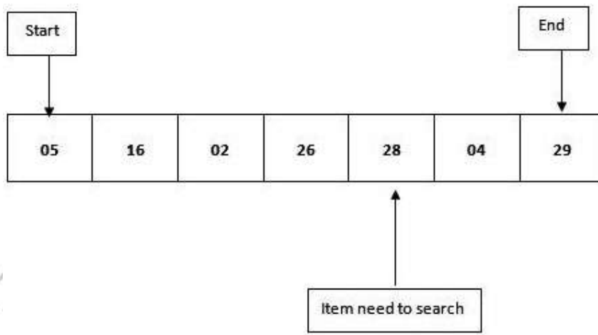
Fig. 16.1 Linear Search
